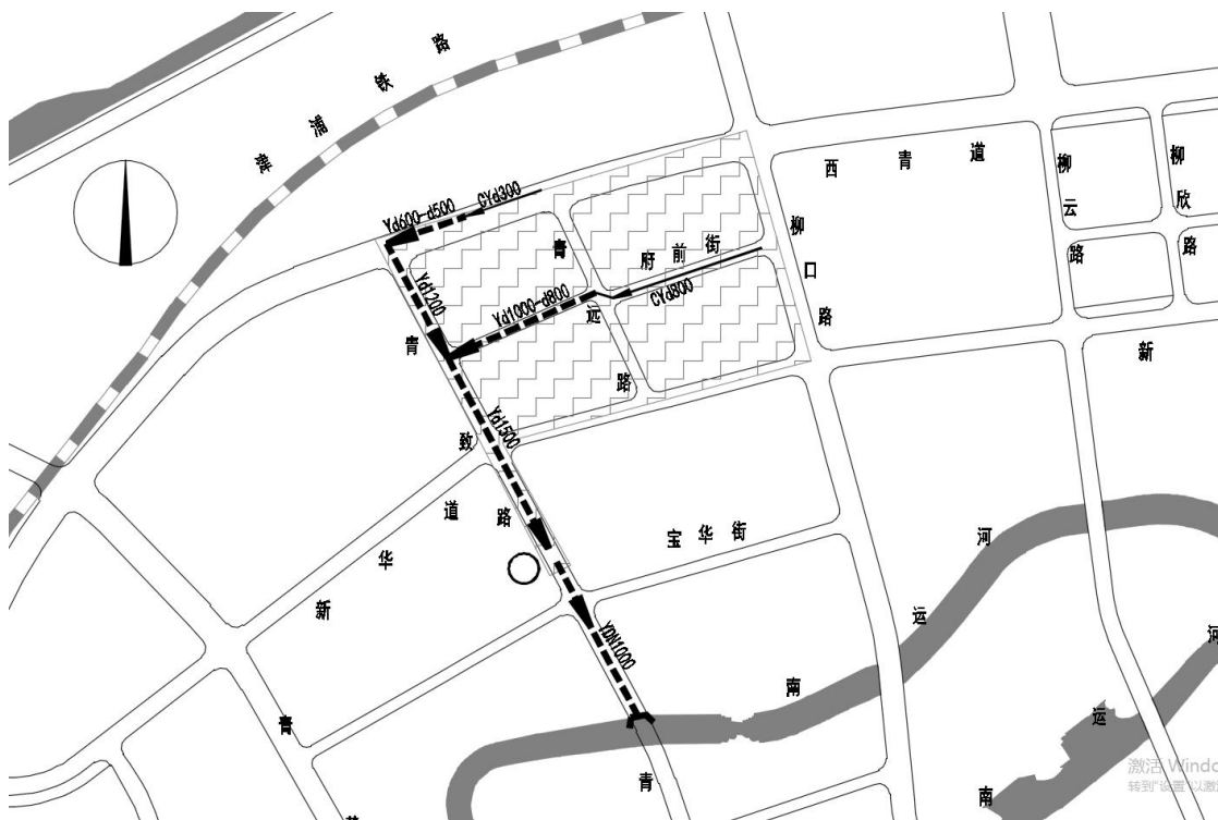
图 1-1 管线平面布置图
